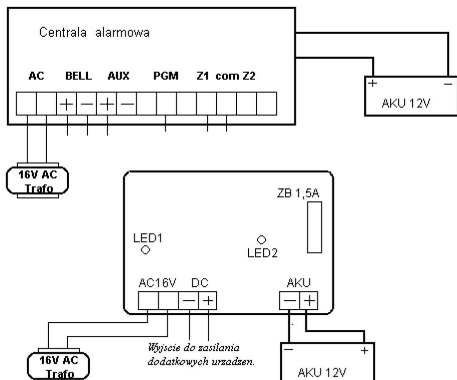
Schemat podłączenia zasilacza buforowego 1,5A
